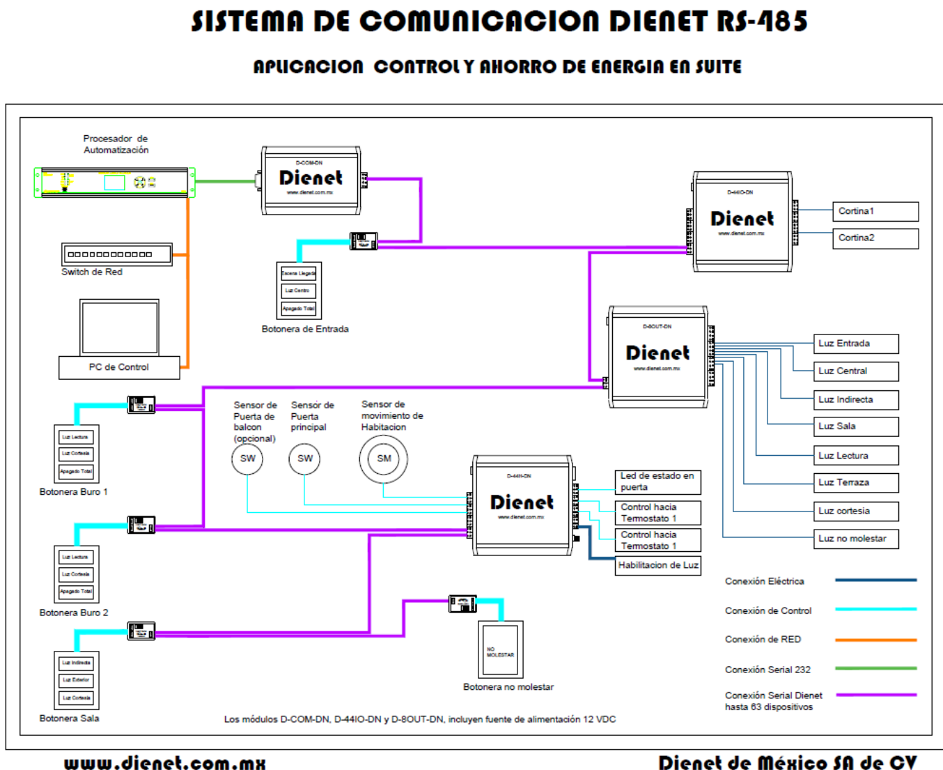
Ilustración 4.-Sistema de Dienet RS485 de Control de Suite
