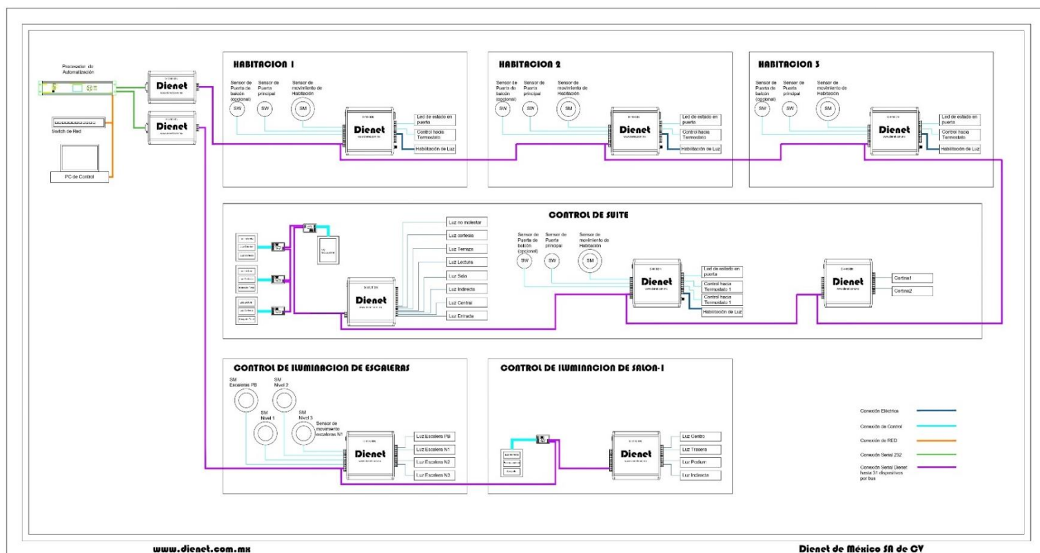
Ilustración 5. –Sistema RS485 Dienet para control de Habitaciones
