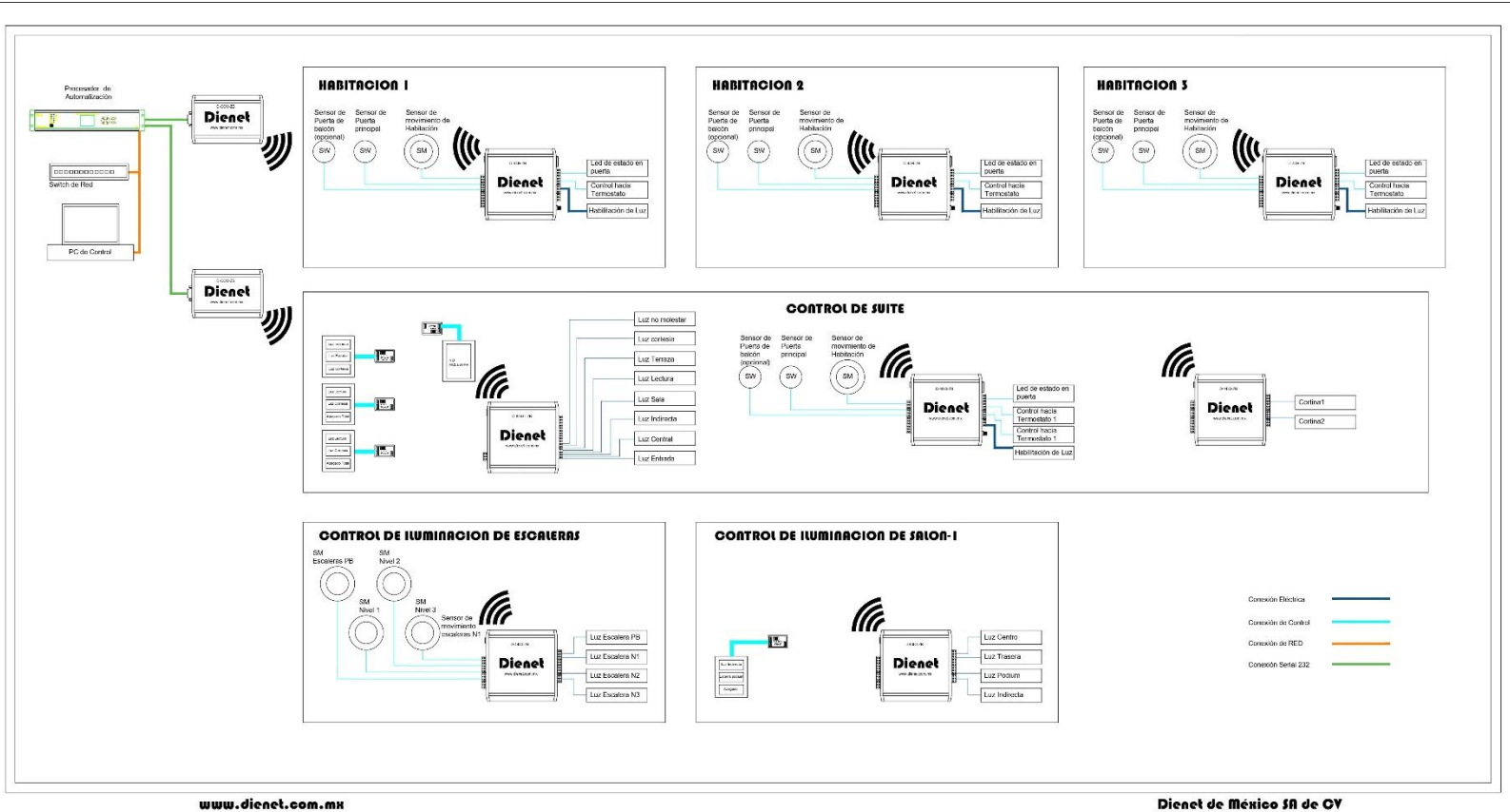
Ilustración 5.-Sistema ZB Dienet para control de Habitaciones
