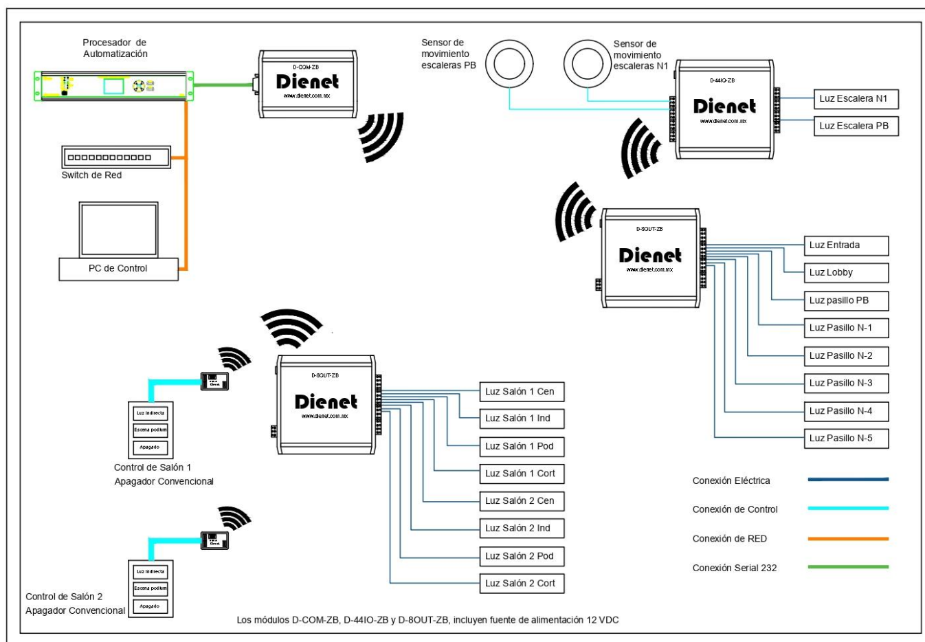
Ilustración 4.-Sistema de Dienet ZB de Control de Suite
